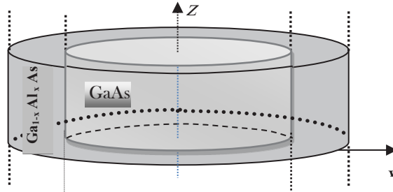
شکل (۱) ساختار یک سیم کوانتومی از GaAs در یک محیط نیمه‌رسانای قطبی Ga_xAl_{1-x}As محصور شده است.
