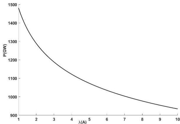
شکل ۱ وابستگی توان بحرانی خودکانونی نسبی به طول موج لیزر.
