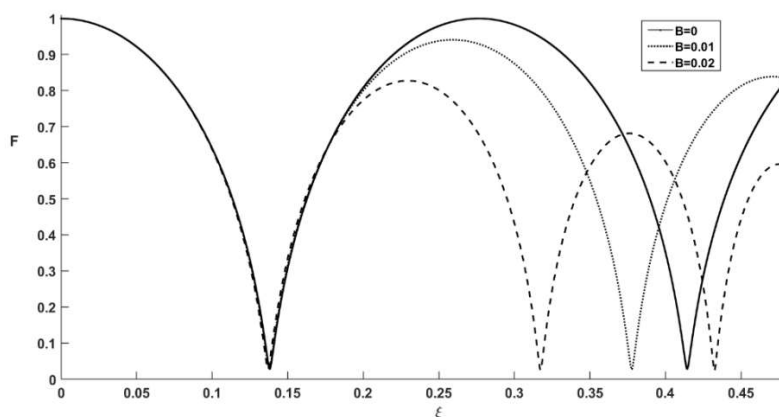
شکل ۲ مقایسه پارامتر پهنای باریکه در سه گرادیان چگالی B=0 (خط ممتد)، B=0.01 (نقطه‌چین)، B=0.02 (خط چین) در پلاسما بی‌برخورد.
