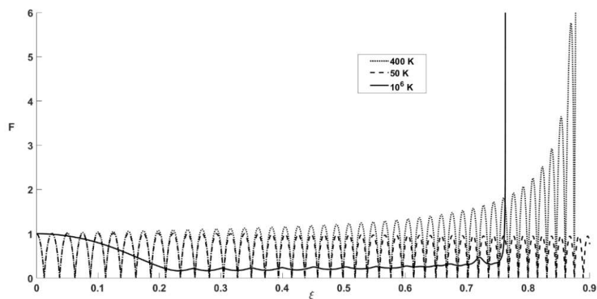
شکل ۵ انتشار باریکه لیزر در پلاسما با دمای ۵۰K (خط چین)، ۴۰۰K (نقطه چین)، ۱۰ ۶ K (خط ممتد).
