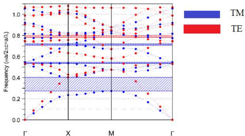
شکل ۱ ساختار نوار بلور فوتونی پایه.
